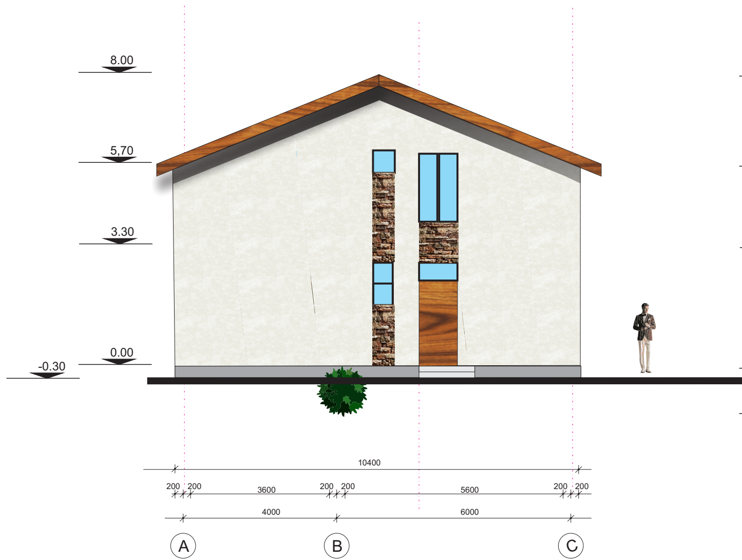
ԲԱԿԱՅԻ ՃԱԿԱՏ A-B ԱՌԱՆՑՔՆԵՐԻ ՄԻՋԵԿ Մ 1:100
