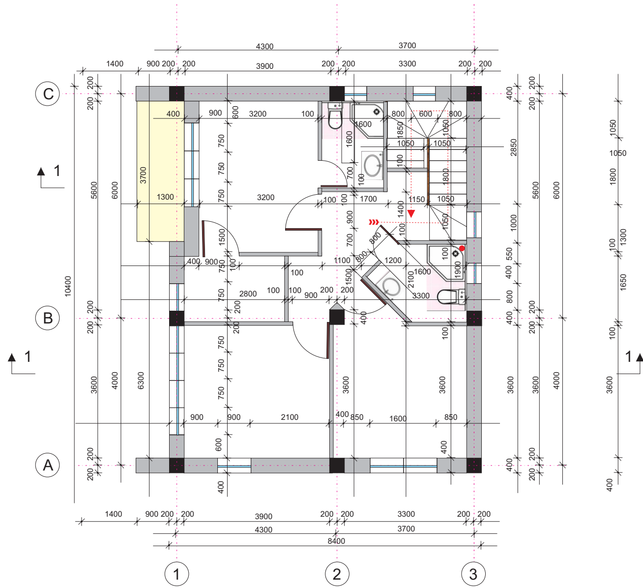
ԵՐԿՈՐԴ ՀԱՐԿԻ ՀԱՏԱԿԱԳԻՃ Մ 1:100
