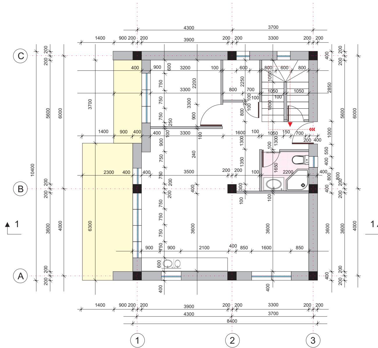
ԱՌԱՋԻՆ ՀԱՐԿԻ ՀԱՏԱԿԱԳԻԾ Մ 1:100
