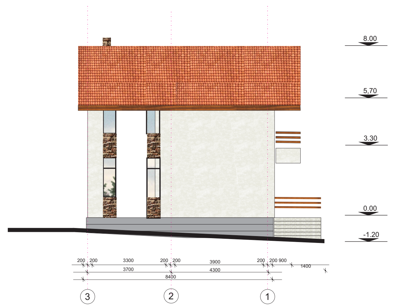
ԿՈՂԱՅԻՆ ՃԱԿԱՏ Բ-Ա ԱՌԱՆՑՔՆԵՐԻ ՄԻՋԵՎ Մ 1:100
