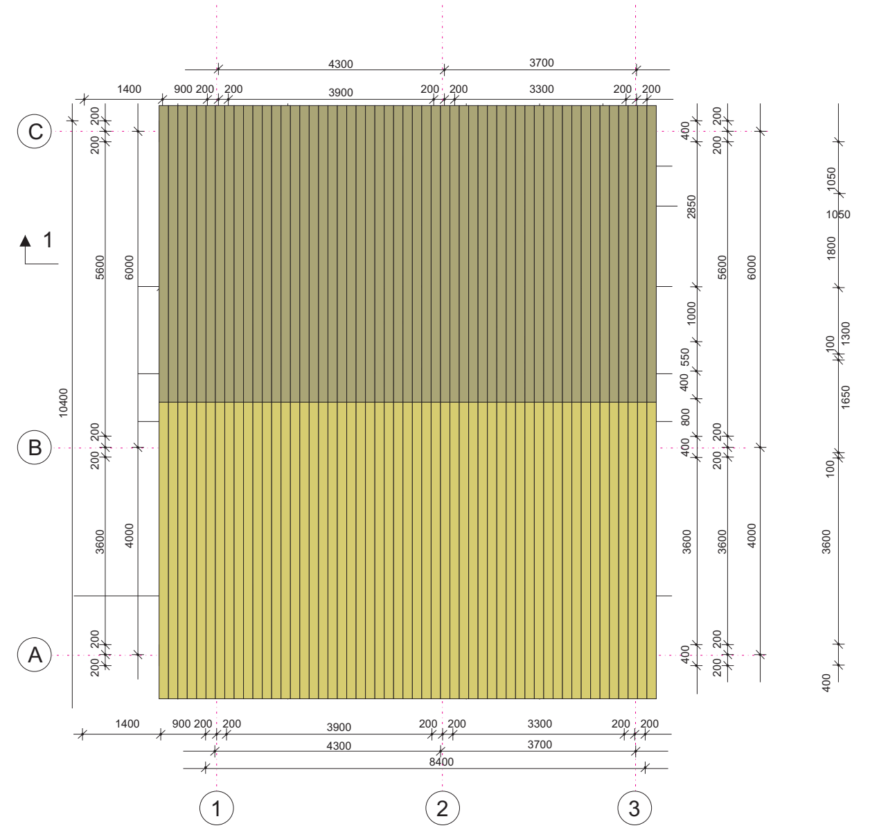
ՏԱՆԻՔԻ ՀԱՏԱԿԱԳԻԾ Մ 1:100
